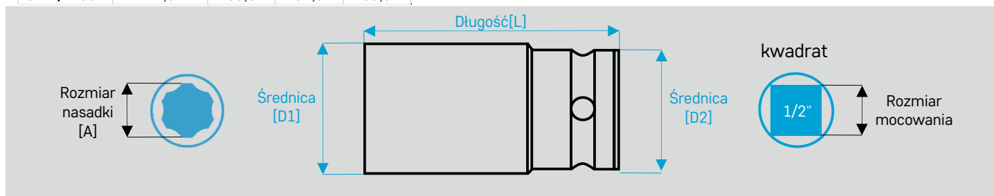
Nasadki udarowe 6-kątne hexagon Surface Drive TORX® PLUS - dłuższa wersja
