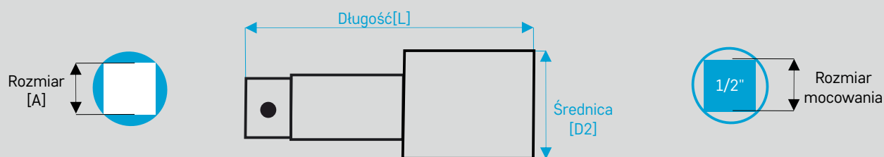
Przedłużka do klucza z kulką
