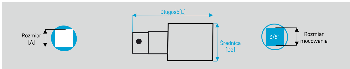
Przedłużka do klucza z kulą
