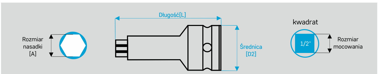
Nasadki wkrętaskowe 6-kątne hexagon
