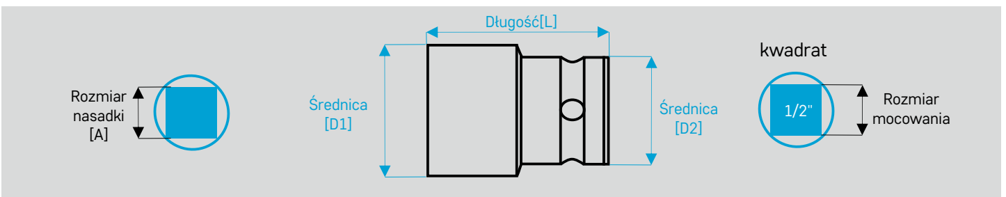
Nasadki udarowe kwadrat
