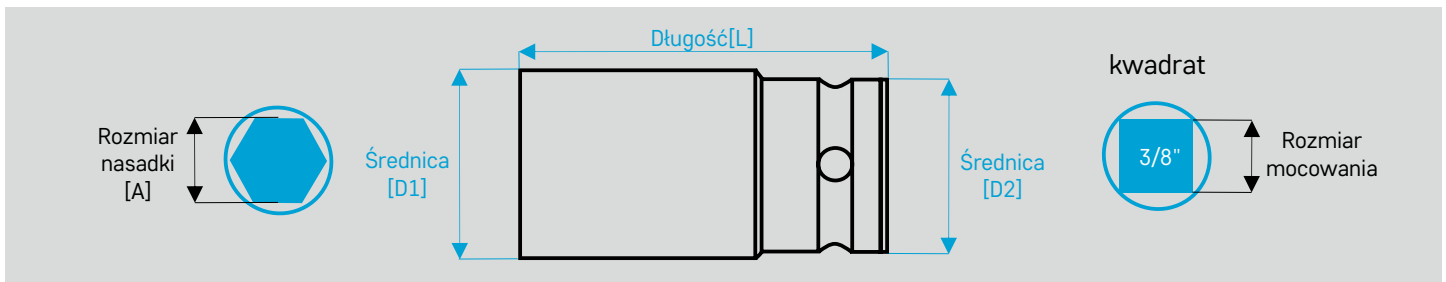
Nasadki udarowe 6-kątne hexagon - dłuższa wersja cienkościenne
