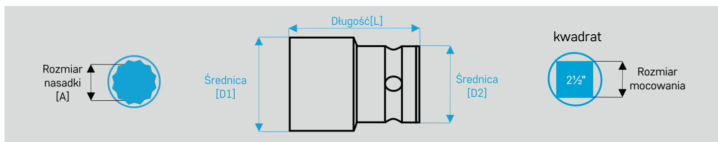
Nasadki udarowe 12-kątne double hexagon
