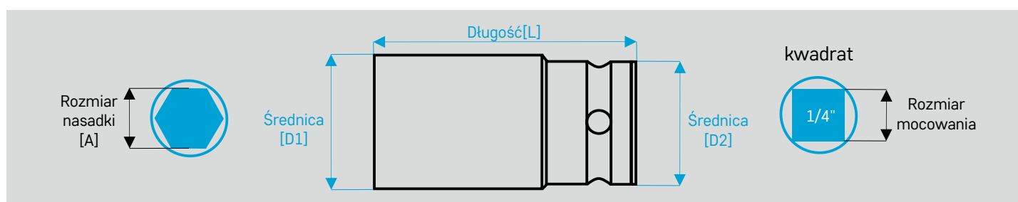
Nasadki udarowe 6-kątne hexagon - dłuższa wersja
