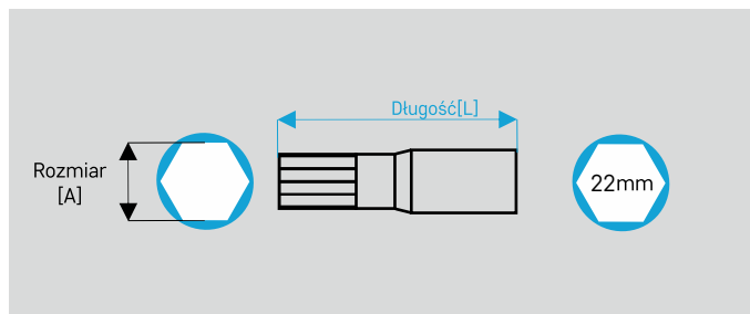
Końcówki imbusowe 22mm
