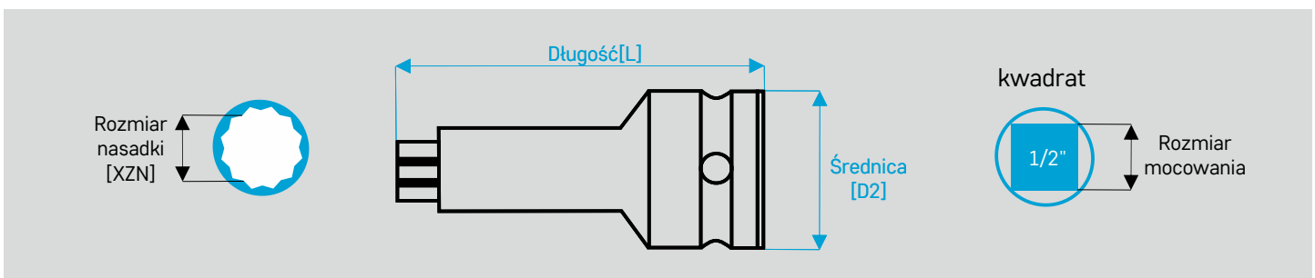
Nasadki wkrętaskowe XZN
