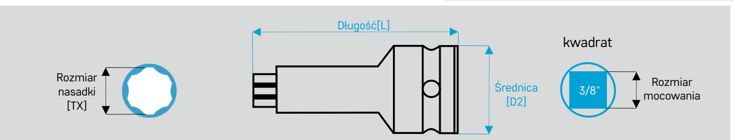
Nasadki wkrętakowe TORX® PLUS socket screws
