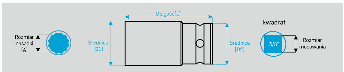
Nasadki udarowe 12-kątne double hexagon - dłuższa wersja
