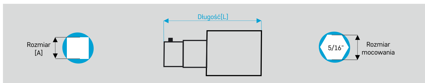
Łącznik do klucza z kątkiem sprężynowym
