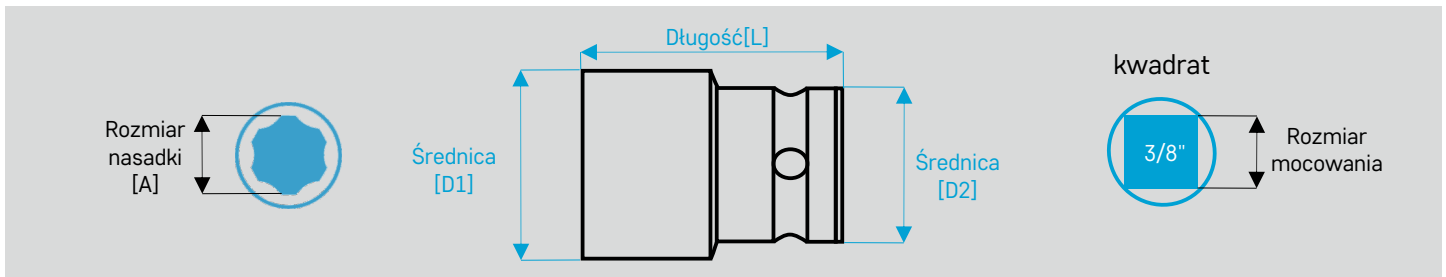
Nasadki udarowe 6-kątne hexagon Surface Drive TORX® PLUS cienkościenne
