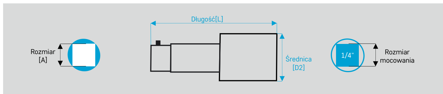
Przedłużka do klucza z kołkiem sprężynowym
