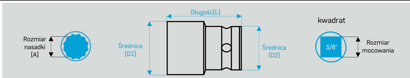
Nasadki udarowe 12-kątne double hexagon - krótka wersja cienkościenne
