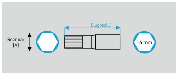
Końcówki imbusowe 16 mm
