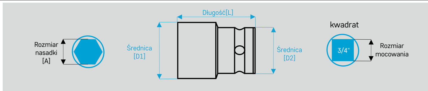
Nasadki udarowe 6-kątne hexagon
