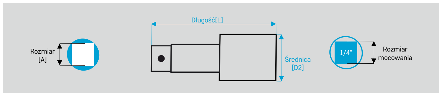
Przedłużka do klucza z kulką
