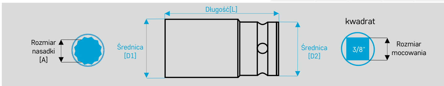
Nasadki udarowe 12-kątne double hexagon - dłuższa wersja cienkościenne
