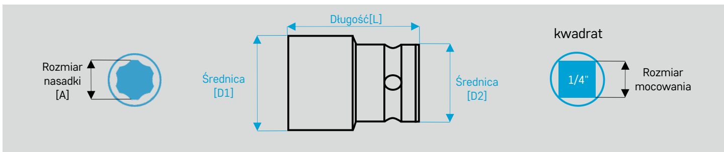
Nasadki udarowe 6-kątne hexagon Surface Drive TORX® PLUS z magnesem
