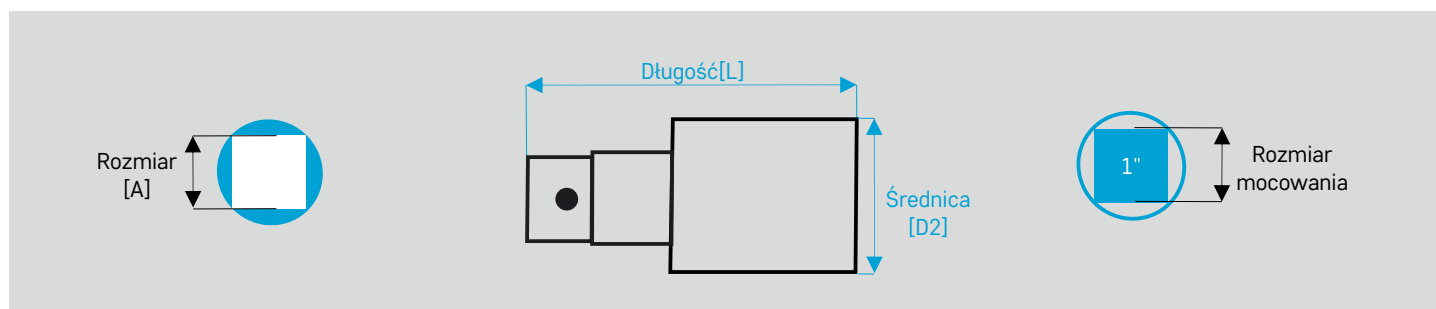
Łącznik do klucza z szybkozłączką, z kulką
