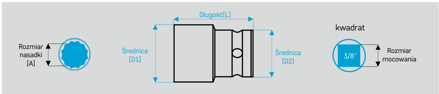
Nasadki udarowe 12-kątne double hexagon
