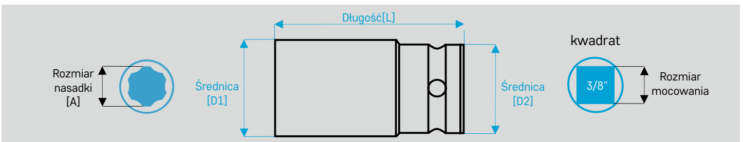
Nasadki udarowe 6-kątne hex. Surface Drive TORX® PLUS cienkościenne - wersja dłuższa
