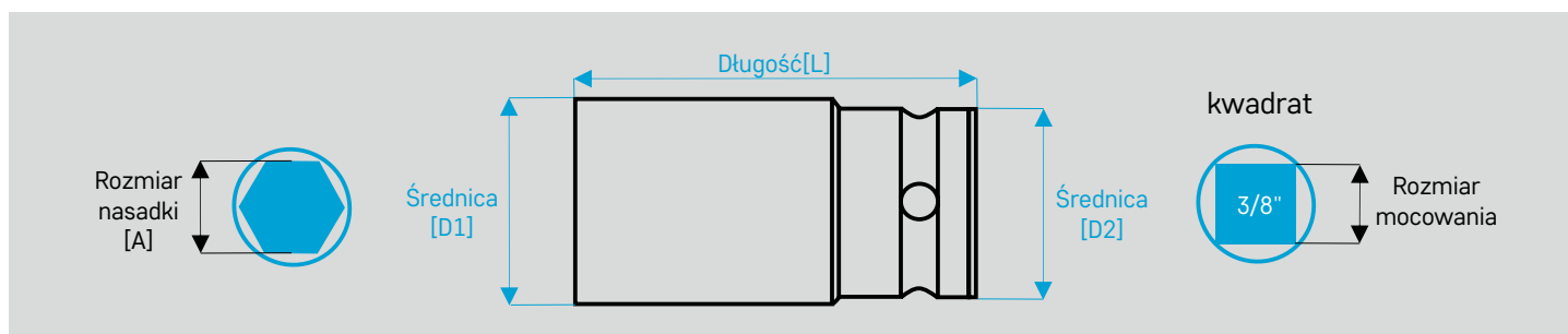
Nasadki udarowe 6-kątne hexagon - dłuższa wersja
