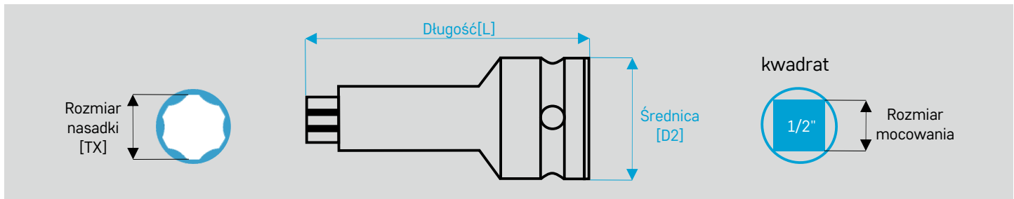
Nasadki wkrętaskowe TORX® PLUS socket screws
