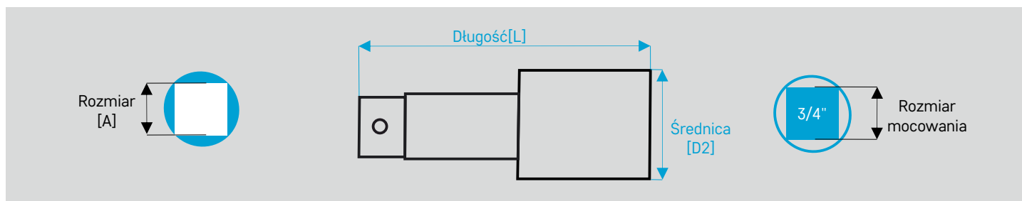
Przedłużka do klucza z otworem przelotowym
