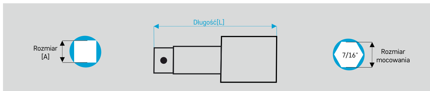
Łącznik do klucza z szybkozłączką, z kulką
