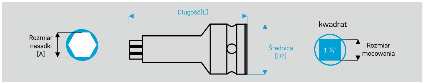
Nasadki wkrętakowe 6-kątne hexagon
