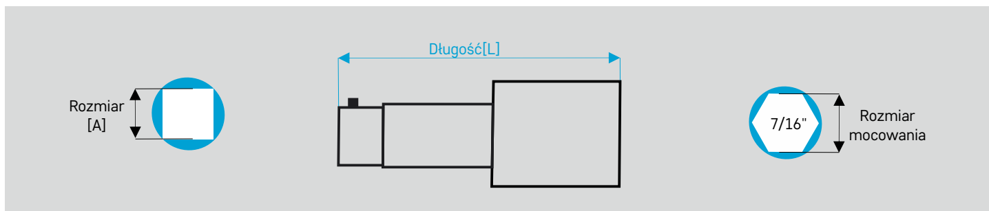
Łącznik do klucza z kołkiem sprężynowym
