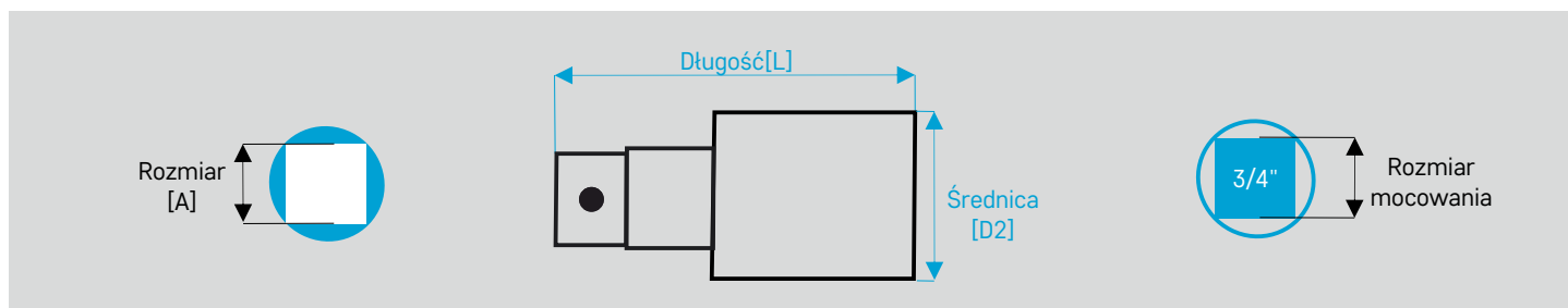
Łącznik do klucza z szybkołączką, z kulką
