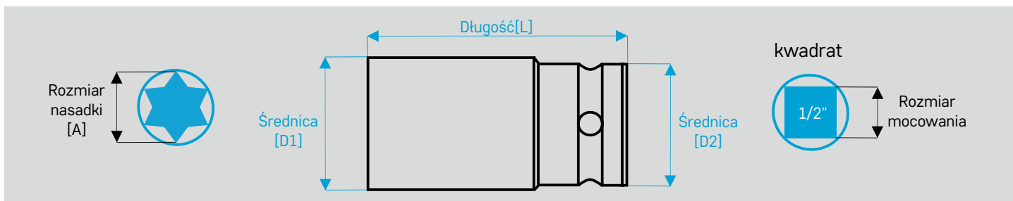
Nasadki udarowe TORX® socket screws - dłuższa wersja
