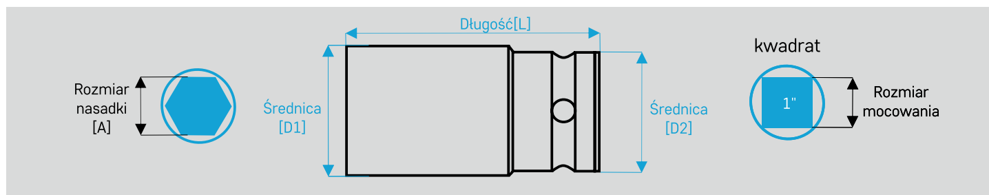
Nasadki udarowe 6-kątne hexagon - dłuższa wersja
