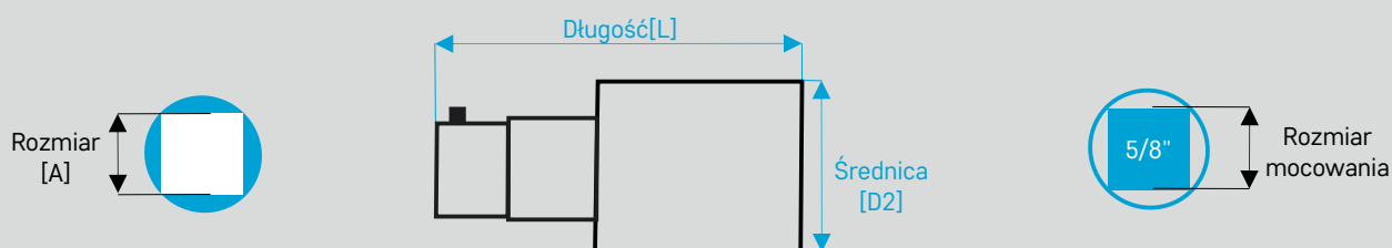
Łącznik do klucza z kotkiem sprężynowym
