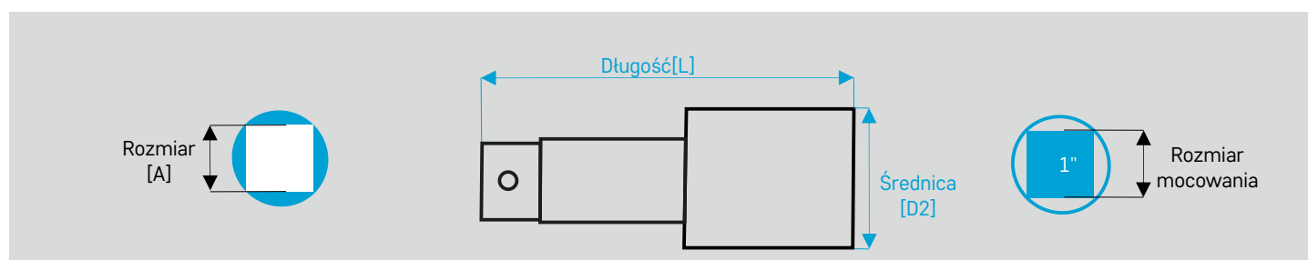
Przedłużka do klucza z otworem przelotowym
