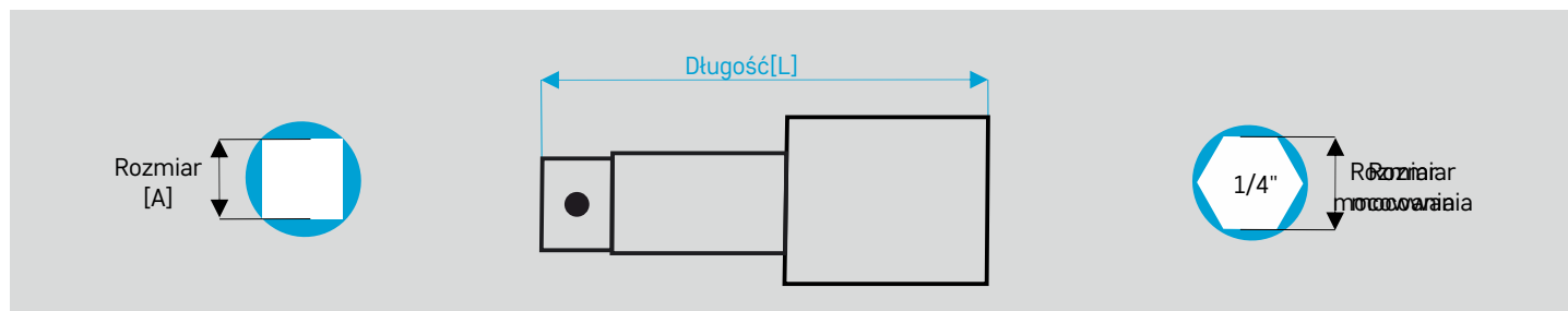
Łącznik do klucza z kulką
