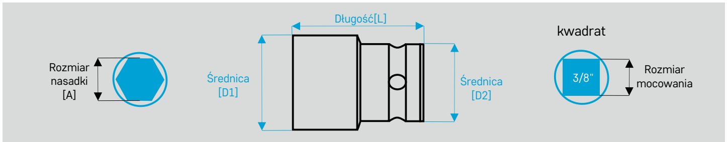
Nasadki udarowe 6-kątne hexagon - krótka wersja cienkościenne
