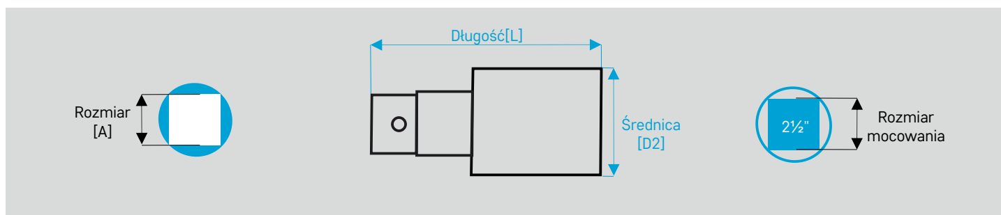
Łącznik do klucza z otworem przelotowym
