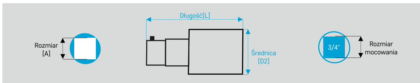
Łącznik do klucza z kołkiem sprężynowym
