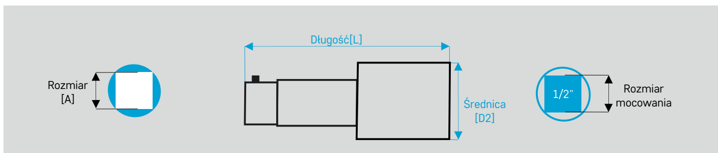
Przedłużka do klucza z kotłkiem sprężynowym
