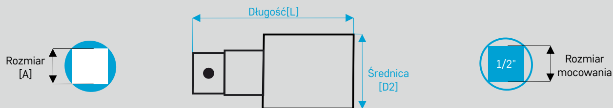
Łącznik do klucza z szybkołączką, z kulką
