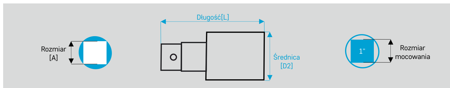
Łącznik do klucza z otworem przelotowym
