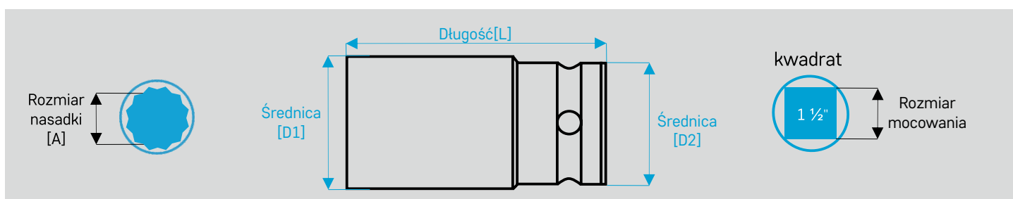
Nasadki udarowe 12-kątne double hexagon - dłuższa wersja
