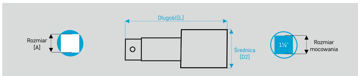
Przedłużka do klucza z otworem przelotowym
