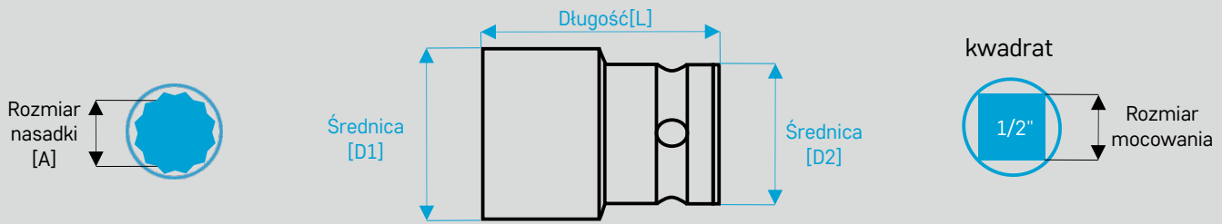
Nasadki udarowe 12-kątne double hexagon
