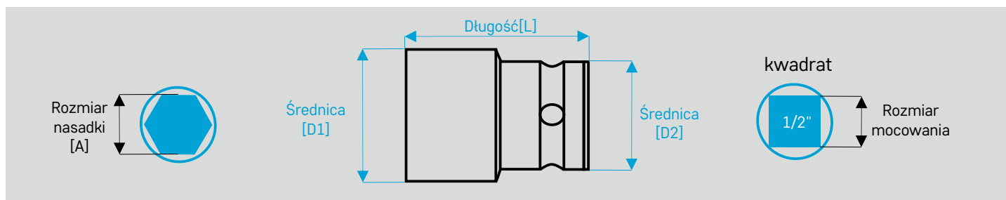
Nasadki udarowe 6-kątne hexagon - krótka wersja cienkościenne
